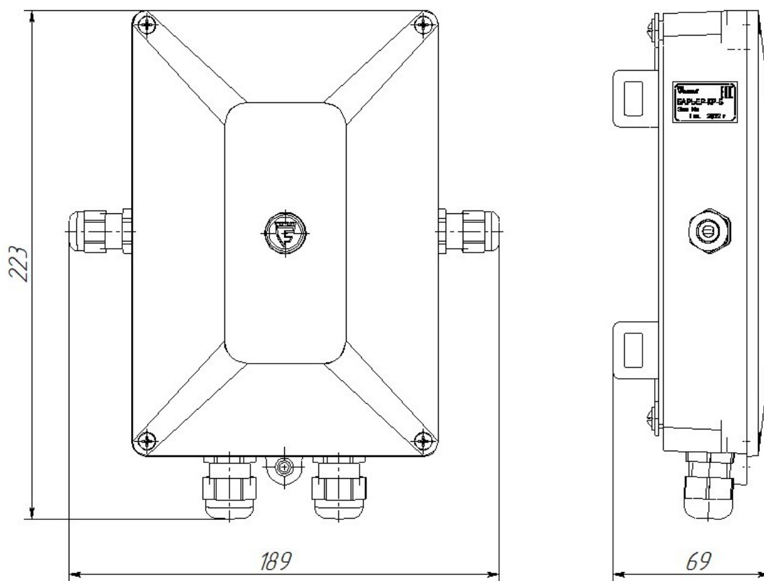
Рисунок 1 – Внешний вид коробки (стандартная комплектация)
